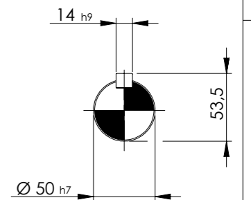
Detalhe eixo de saída Output shaft detail Detalle eje de salida (sem escala/nó scale/sin escala)
