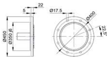
Flange Ø 450
