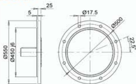
Flange Ø 550
